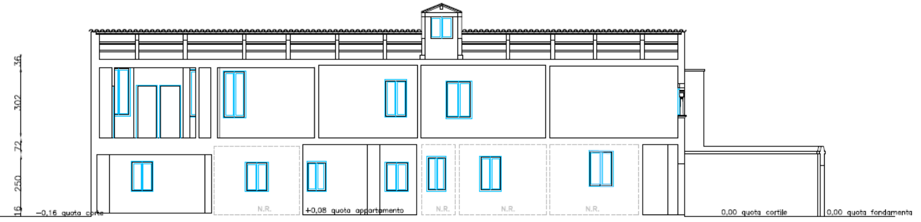
SEZIONE A-A'
