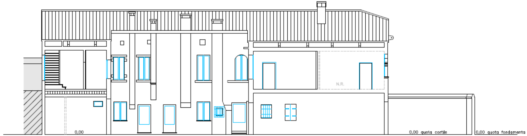
SEZIONE B-B'
