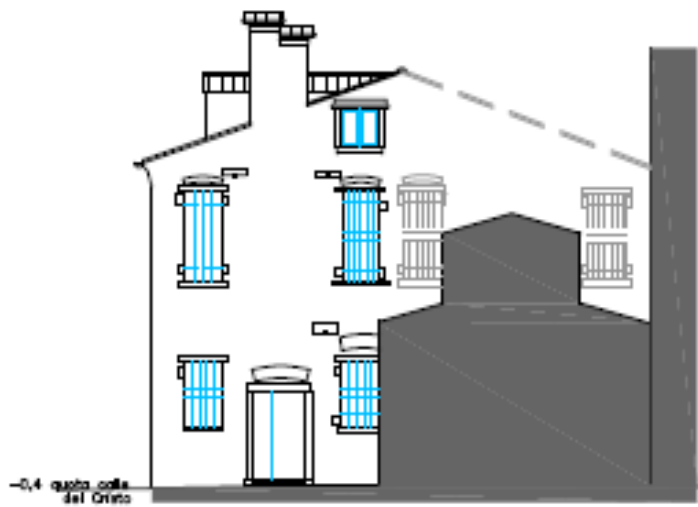
PROSPETTO NORD
